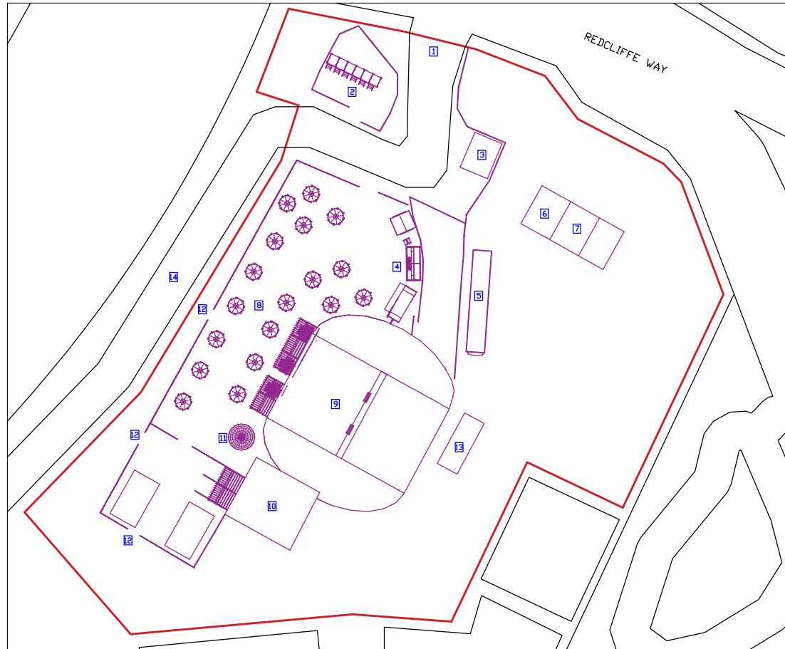
SITE PLAN (1:500)
